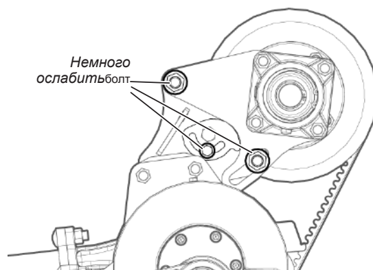
Рис. 161 - Натяжение ремня ножей: ослабление стопорной гайки и болта.
