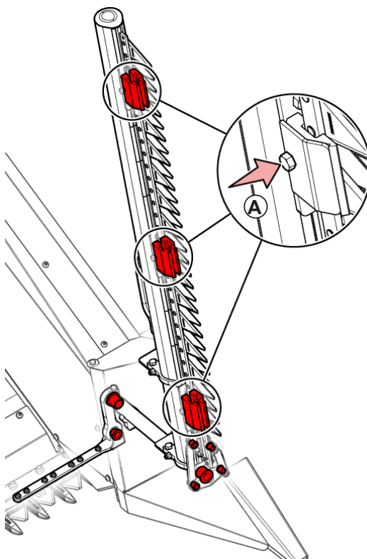
Рис. 93 - Места техобслуживания вертикальных ножниц.
