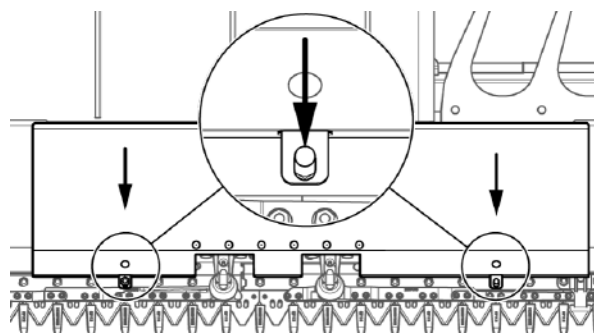
Рис. 220 - Пластина головки ножа
