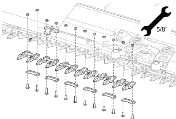
Рис. 226 - Снятие защитных устройств, которые окружают головку правого ножа
