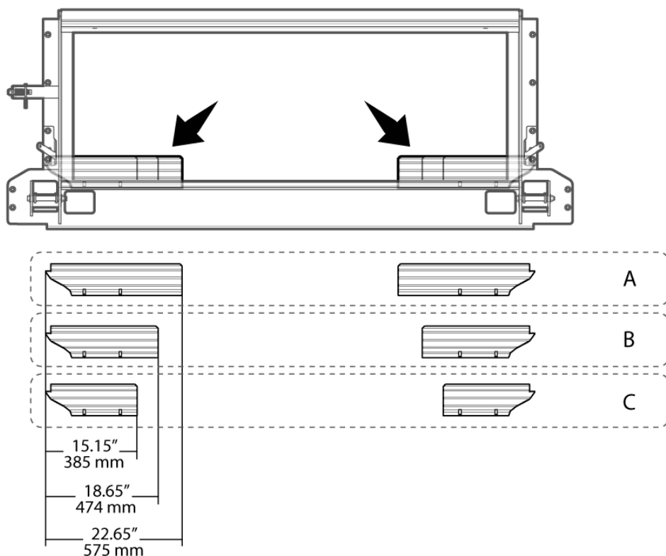
Рис. 303 - Гнездо AGCO - Схема 2
