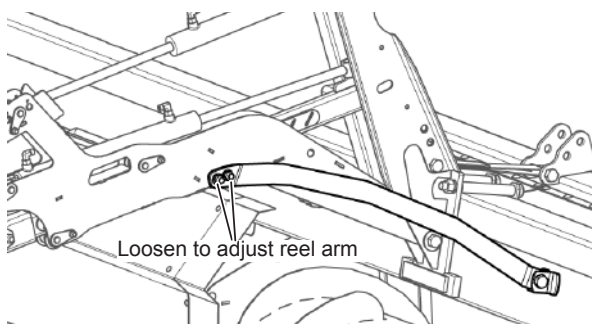
Рис. 75 - Центрирование мотовила — кронштейн центрального луча мотовила
