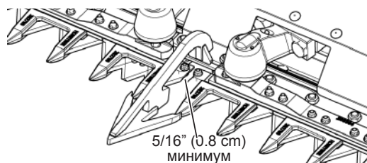
Рис. 219 - убедитесь что два ножа не касаются друг друга во время работы
