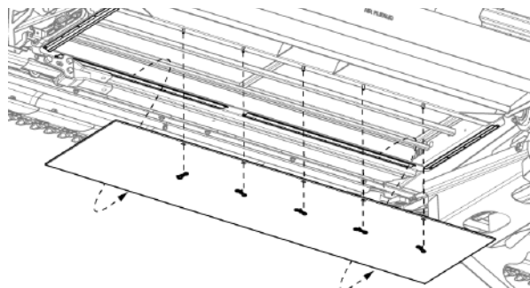
Рис. 189 - Снятие панели очистного люка центрального полотненного транспортера.
