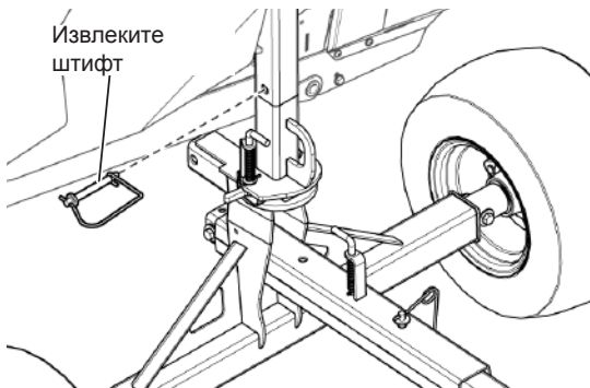
Рис. 48 - Извлечение штифта сцепного устройства передней тележки.
