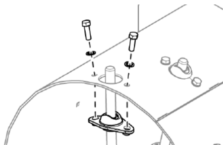
Рис. 257 - Замена направляющих устройств для пальцев подающего шнека.
