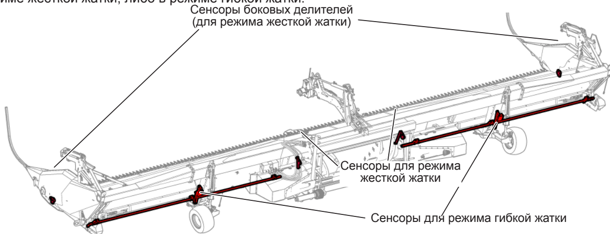
Рис. 306 - Места расположения сенсоров системы контроля высоты жатки.
