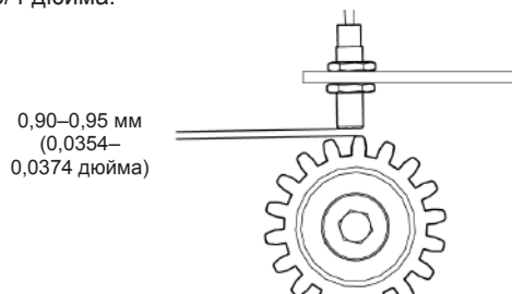
Рис. 196 - Регулировка сенсора скорости вращения мотовила.
