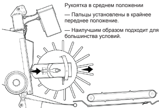
Рис. 76 - Пальцы барабана подающего шнека в среднем положении.
