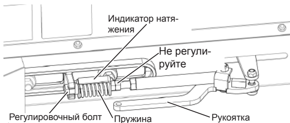
Рис. 178 - Регулировка натяжения полотенного транспортера
