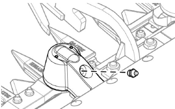
Рис. 225 - Временно снимите тавотницу
