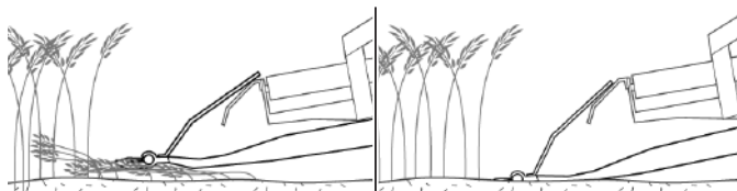
Рис. 125 - Слишком низкое давление воздуха в режиме гибкой жатки: режущий защитный экран зарывается в почву. Рис. 124 - Слишком высокое давление воздуха в режиме гибкой жатки: режущий аппарат движется над растениями.
