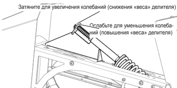
Рис. 252 - Регулировка параметров колебаний пружин боковых делителей.
