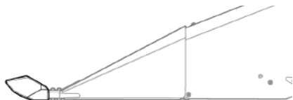
Рис. 118 - Усеченная насадка для бокового делителя
