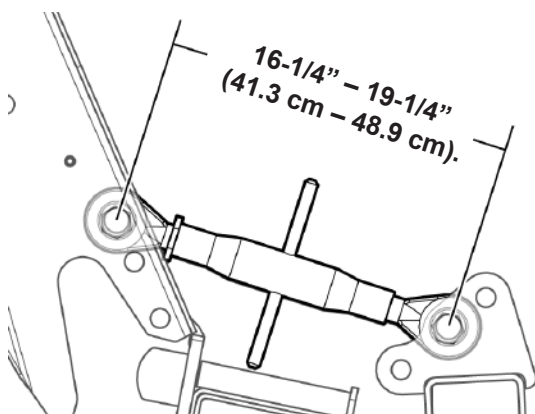
Рис. 111 - Использование режима наклона жатки
