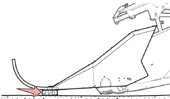
Рис. 66 - Деревянный блок, подложенный под делители.
