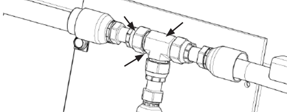
Рис. 273 - Проверка Т-образных фитингов, расположенных перед подкосами на предмет утечек
