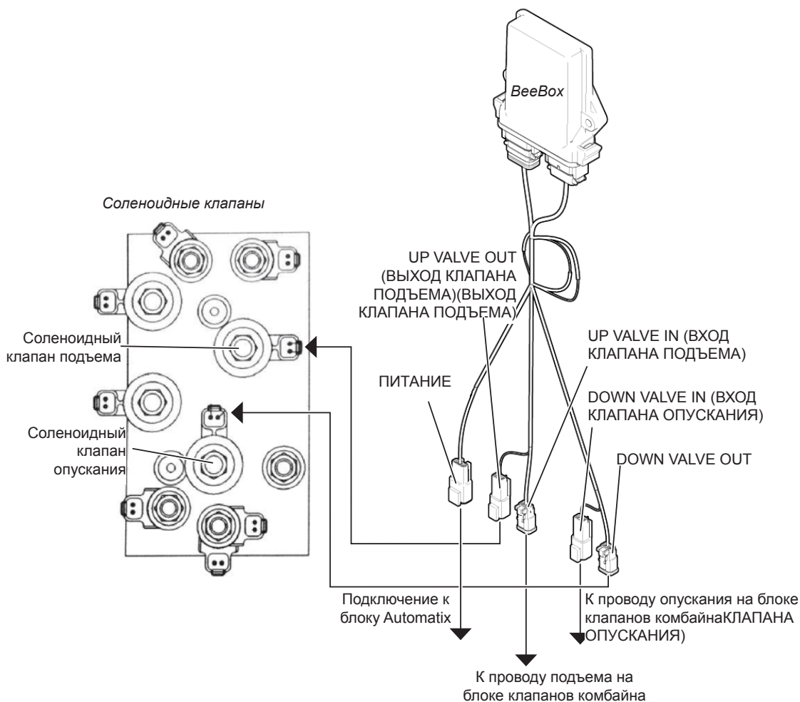
Рис. 309 - Устройство BeeBox, предназначенное для использования на комбайнах с двухпозиционными распределительными клапанами.
