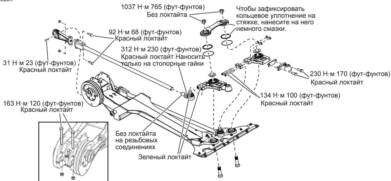
Рис. 216 - Рекомендуемые значения моментов затяжки компонентов привода ножей (подробные сведения см. в разделе разделе 22.8 на стр. 165)
