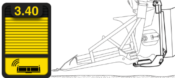
Рис. 143 - Панель оперативных данных - полный диапазон движения жатки доступен
