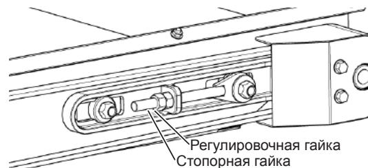
Рис. 182 - Регулировка натяжения центрального полотенного транспортера.
