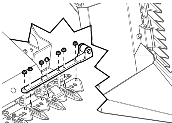
Рис. 92 - Вертикальные ножницы
