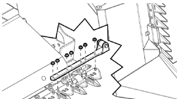
Рис. 96 - Установите головку ножа вертикальных ножниц
