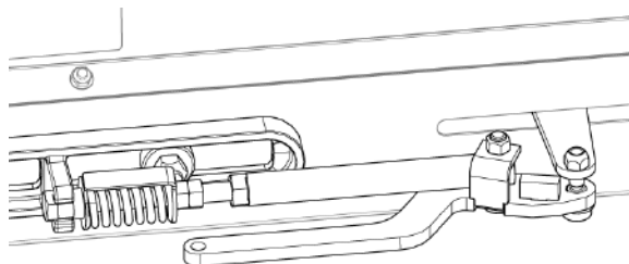
Рис. 108 - Правильное положение рукоятки натяжения полотенного транспортера.
