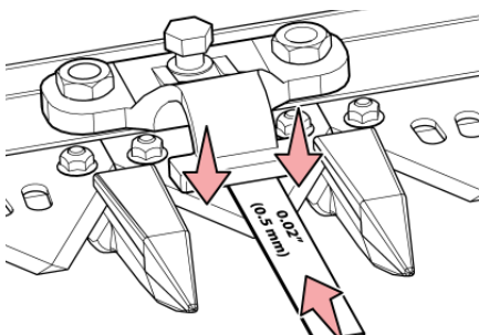
Рис. 238 - Надавите на режущую секцию и вставьте измерительный щуп
