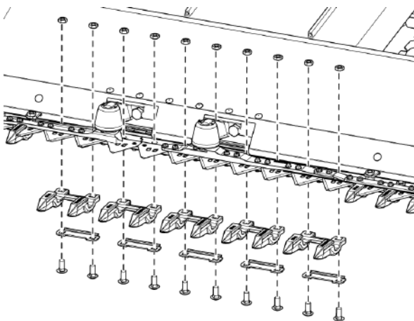
Рис. 241 - Снимите 5 пять центральных защитных щитков
