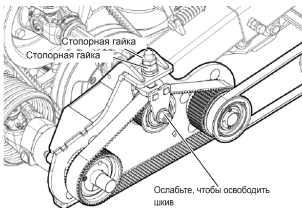
Рис. 173 - Регулировка натяжения первого ремня правого полотенного транспортера
