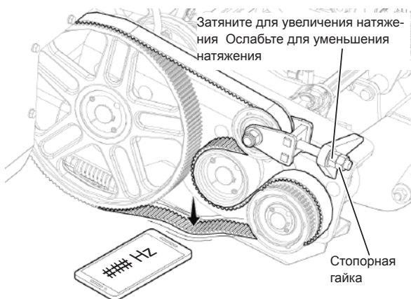
Рис. 154 - Натяжение приводного ремня подающего шнека.
