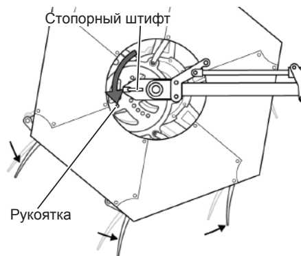
Рис. 114 - Увеличение агрессивности пальцев
