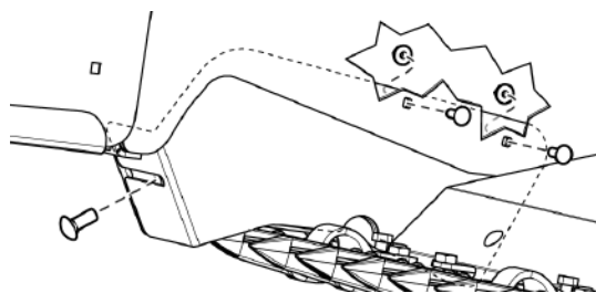
Рис. 245 - Установите привинчивающийся щиток
