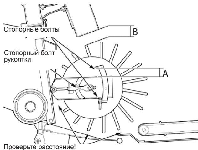
Рис. 78 - Расстояния между барабаном подающего шнека и другими компонентами оборудования.
