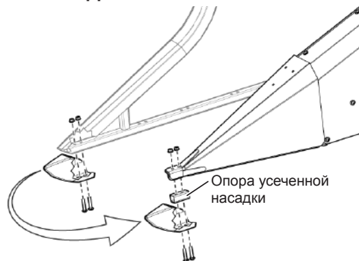
Рис. 251 - Усеченная насадка для бокового делителя.
