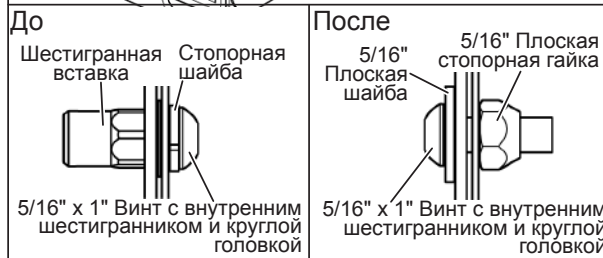
Рис. 100 - Замените шестигранную вставку при необходимости
