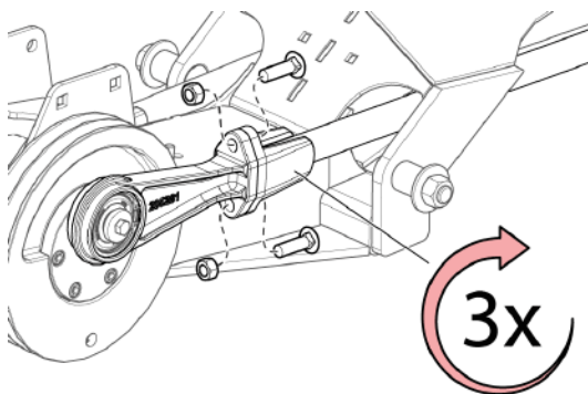
Рис. 218 - Затяните правый рычаг привода ножа на 3 оборота
