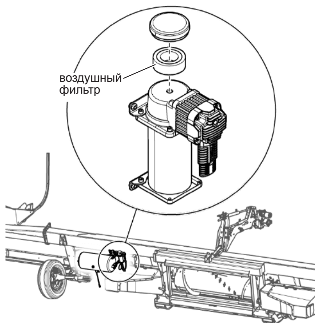
Рис. 275 - Впускной воздушный фильтр воздушного компрессора
