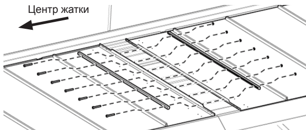
Рис. 184 - Установка соединительного стержня полотенного транспортера.
