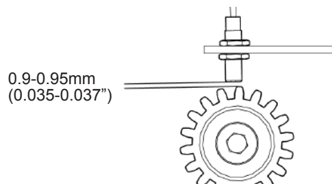
Рис. 148 - Расстояние от сенсора скорости до соответствующей поверхности.
