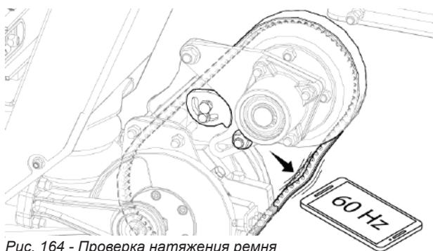
Рис. 164 - Проверка натяжения ремня
