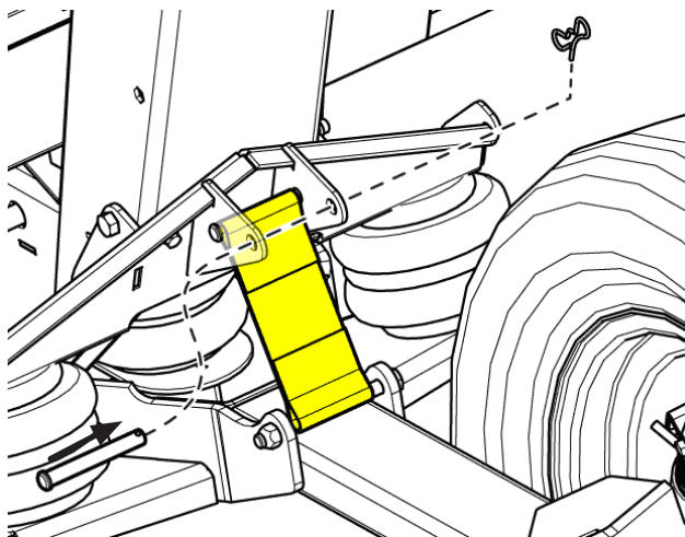
Рис. 57 - Опорный ремень в рабочем положении
