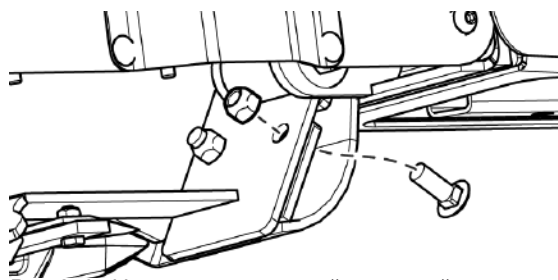
Рис. 246 - Установите концевой кронштейн ползка лопасти
