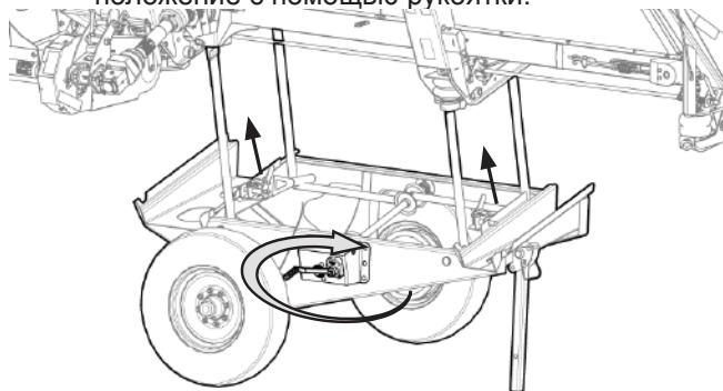
Рис. 284 - Установка транспортной тележки для жатки
