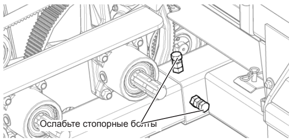
Рис. 168 - Стопорные болты первого приводного ремня левого полотенного транспортера.
