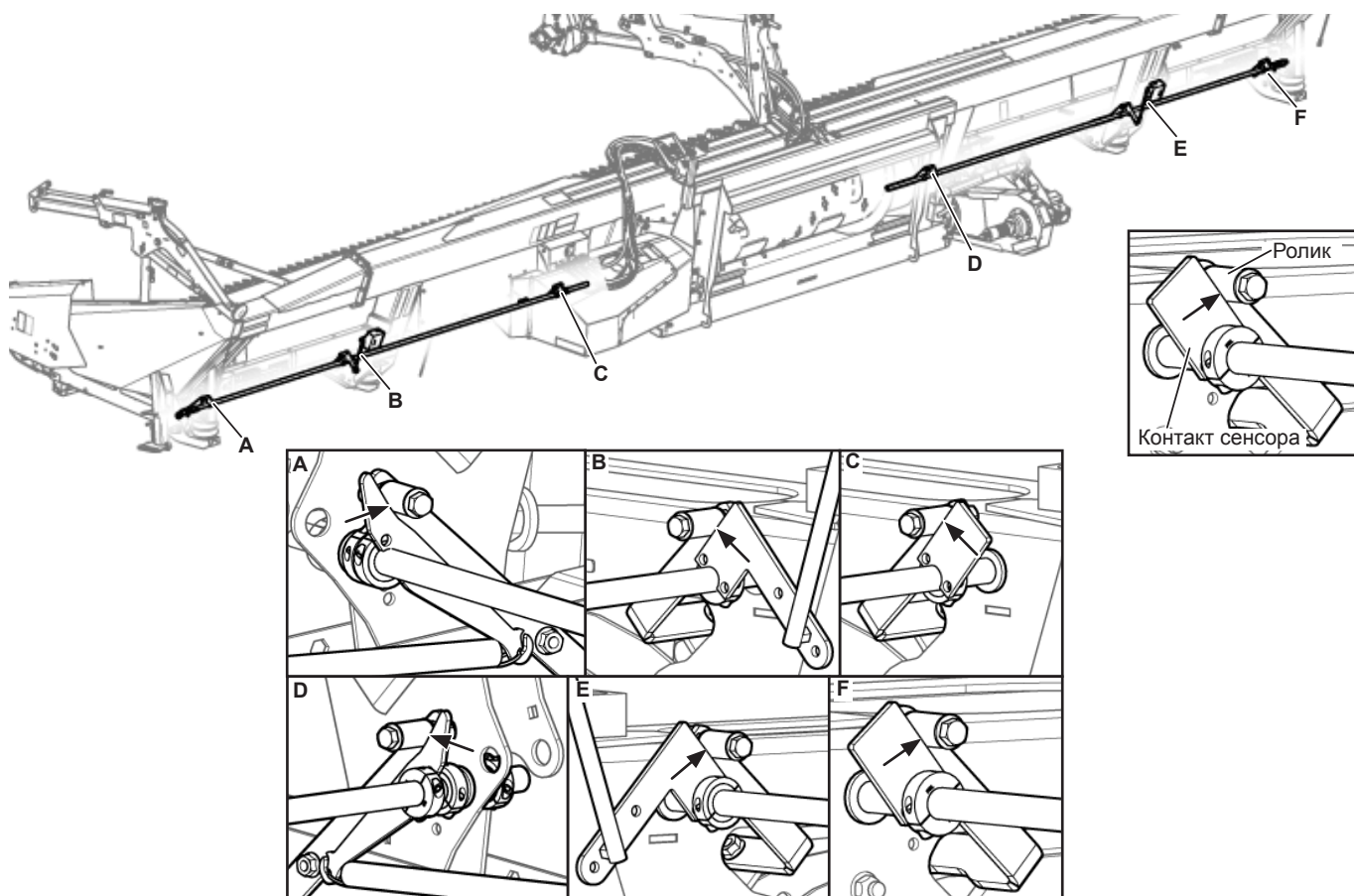
Рис. 265 - Места расположения контактов сенсоров системы контроля высоты гибкой жатки.
