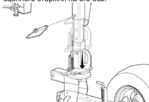
Рис. 286 - Опускание скобы сцепного стержня на ось сцепного стержня
