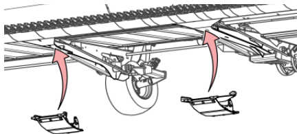
Рис. 81 - Опорные лапы – установленные в месте транспортной тележки
