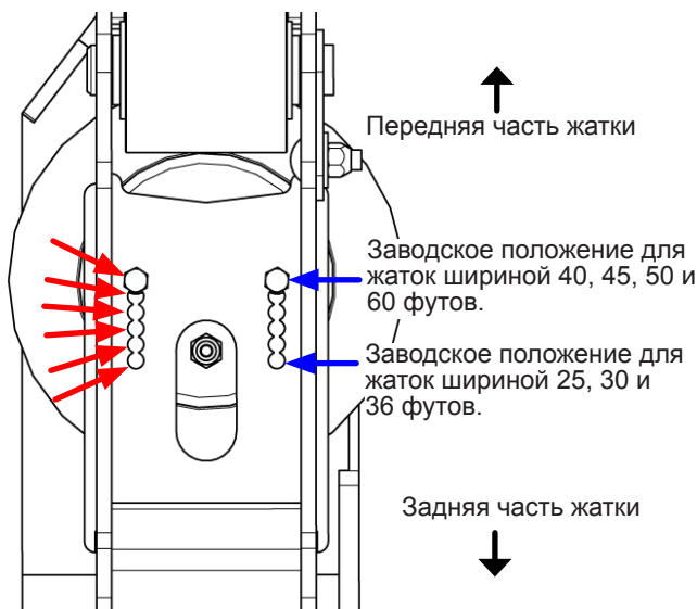
Рис. 276 - Положения воздушных подушек подрамника (показана верхняя часть воздушной подушки)
