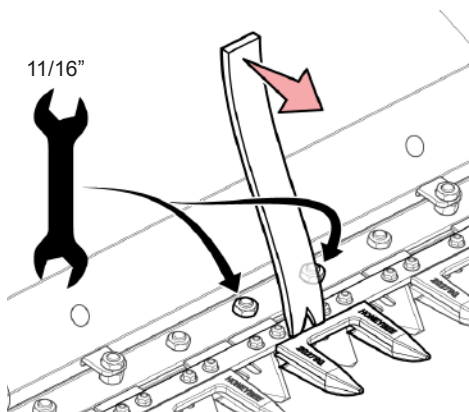
Рис. 222 - Смещайте сдвоенный палец вперед во время затяжки крепежных деталей
