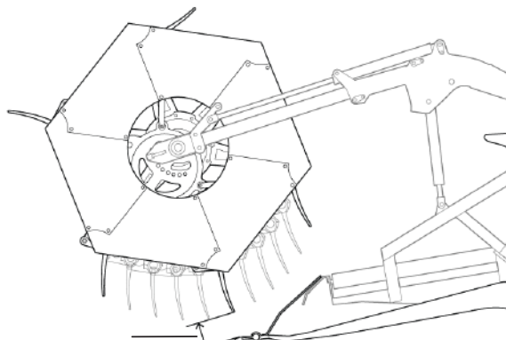
Рис. 112 - Расстояние между пальцами мотовила и режущим аппаратом.
