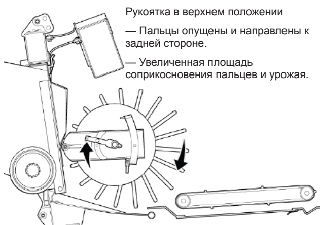
Рис. 77 - Пальцы барабана подающего шнека в нижнем положении
