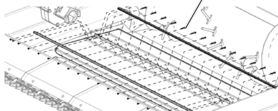
Рис. 191 - Закрепление полотненного транспортера с помощью соединительных стержней.
