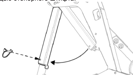
Рис. 194 - Ограничитель хода луча мотовила
