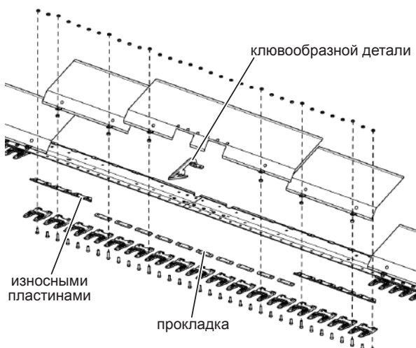
Рис. 221 - Компоновка низкопрофильной режущей системы
