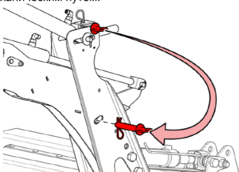
Рис. 195 - Стопорный штифт центрального луча мотовила
