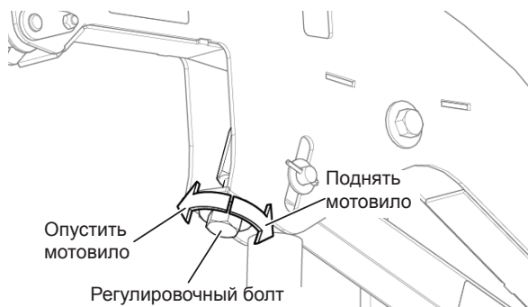
Рис. 70 - Болт для регулировки высоты мотовила.
