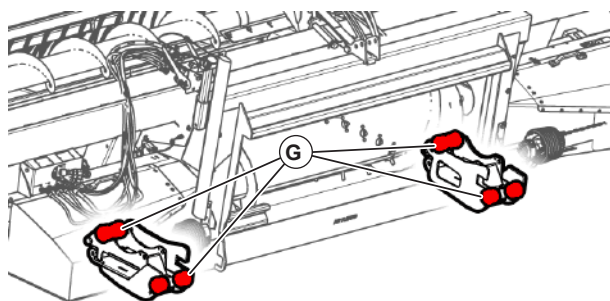
Рис. 305 - Места расположения долговечных втулок
