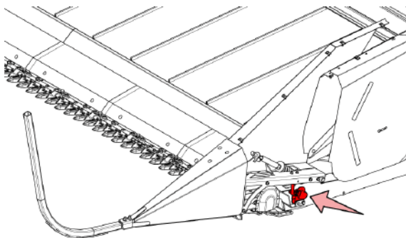
Рис. 268 - Расположение сенсоров делителей
