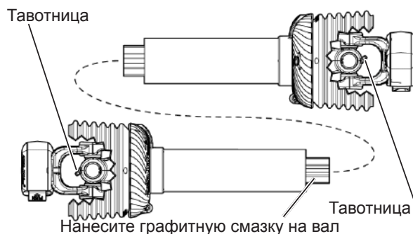
Рис. 263 - Точки нанесения смазки на приводной вал.
