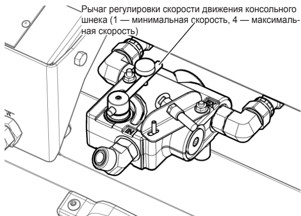
Рис. 90 - Устройство контроля потока урожая (регулятор скорости движения консольного шнека).
