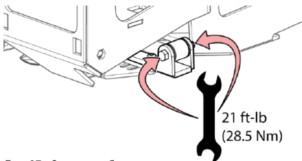
Рис. 97 - Затяните болт головки ножа
