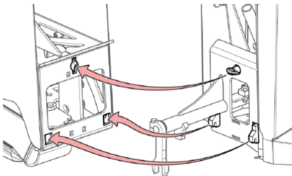
Рис. 103 - Установите узел вертикальных ножниц
