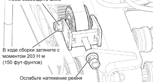
Рис. 167 - Регулировка приводного ремня подающего шнека
