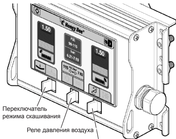
Рис. 137 - Расположение физических переключателей
