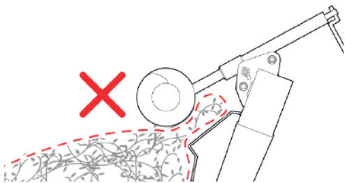
Рис. 89 - Наматывание растений на консольный шнек
