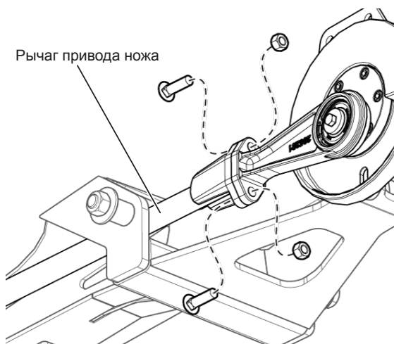
Рис. 217 - Отсоединения обоих рычагов привода ножа
