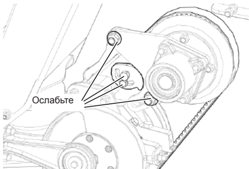
Рис. 166 - Ослабление стопорных механизмов.
