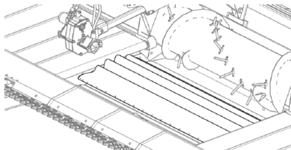
Рис. 190 - Развертывание нового полотненного транспортера на центральной деке.
