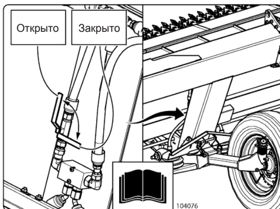
Рис. 121 - Запорный клапан копирующего колеса
