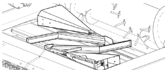
Рис. 282 - Размещение боковых делителей на центральном полотенном транспортере.
