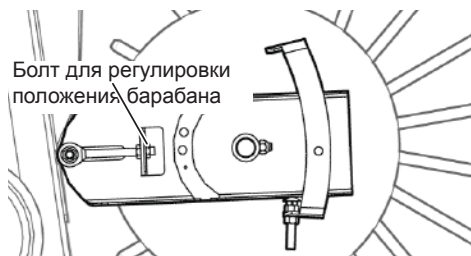
Рис. 254 - Положение барабана подающего шнека.
