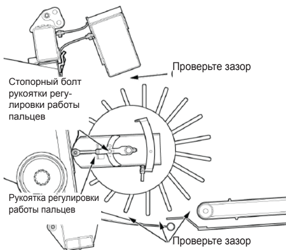
Рис. 253 - Расстояния между барабаном подающего шнека и другими элементами жатки
