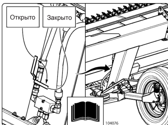
Рис. 64 - Запорный клапан копирующего колеса
