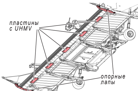
Рис. 86 - Комплект для бездорожья
