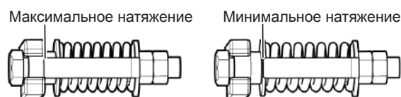
Рис. 179 - Положение индикатора натяжения
