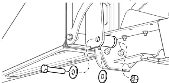
Рис. 243 - Блокировка делителей болтом
