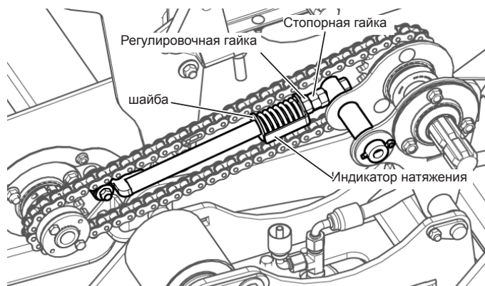
Рис. 174 - Регулировка натяжения приводной цепи центрального транспортера
