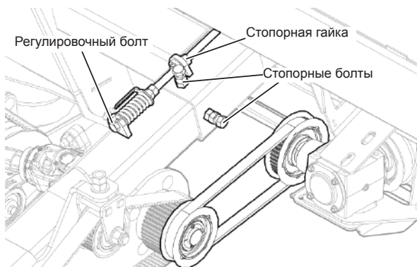
Рис. 159 - Натяжение первого ремня правого полотенного транспортера.
