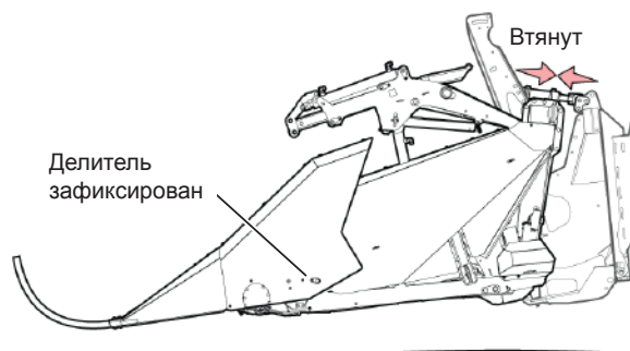
Рис. 67 - Жатка наклонена назад, а делитель зафиксирован.
