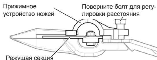
Рис. 79 - Регулировка расстояния между прижимным устройством и режущей секцией
