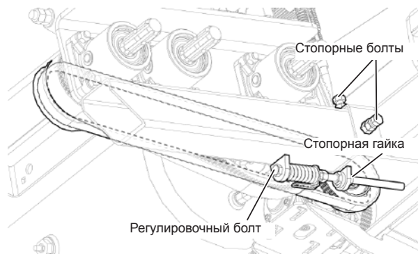
Рис. 155 - Регулировка натяжения первого приводного ремня левого полотенного транспортера.
