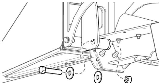
Рис. 101 - Зафиксируйте делитель
