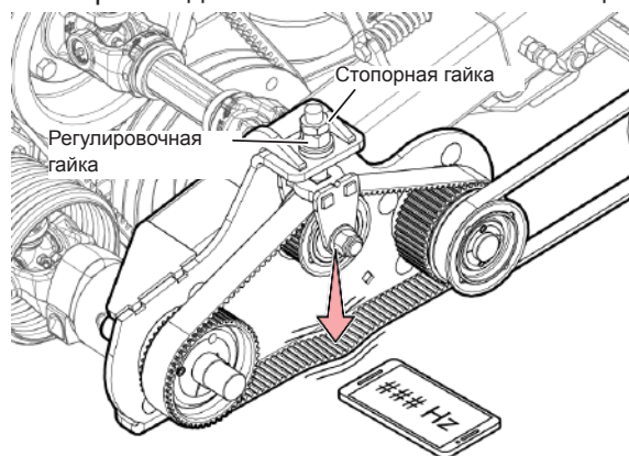
Рис. 158 - Натяжение ремня правого привода
