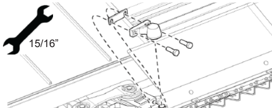
Рис. 230 - Снятие корпуса подшипников с головки левого ножа
