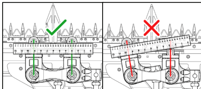
Рис. 215 - Расстояние отрегулировано правильно: угловые рычаги выровнены
