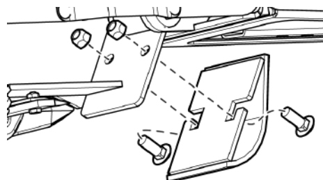
Рис. 244 - Снимите концевой кронштейн ползка лопасти
