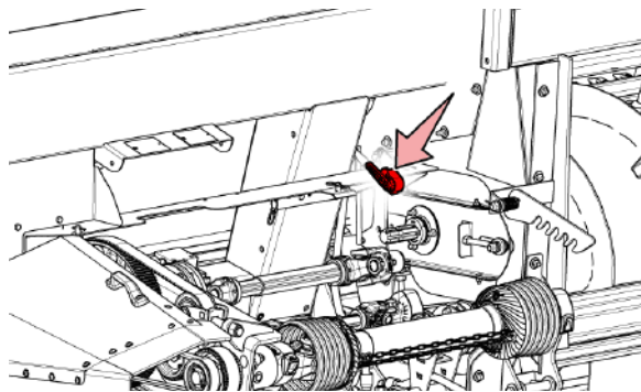
Рис. 270 - Расположение сенсора подрамника
