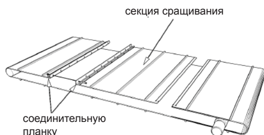
Рис. 193 - сращивания полотенного транспортера
