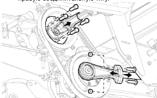
Рис. 165 - Отсоединение соединительной тяги и механизма отбора мощности.
