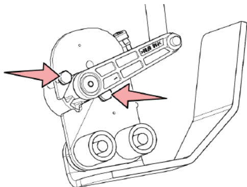
Рис. 269 - Регулировка сенсора делителей
