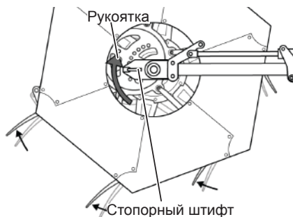
Рис. 113 - Уменьшение агрессивности пальцев
