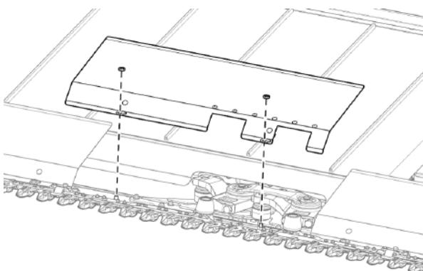
Рис. 224 - Снятие перьевой пластины, расположенной над подшипниками ножей.
