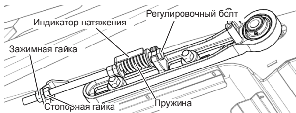
Рис. 183 - Настройка натяжения центрального полотенного транспортера
