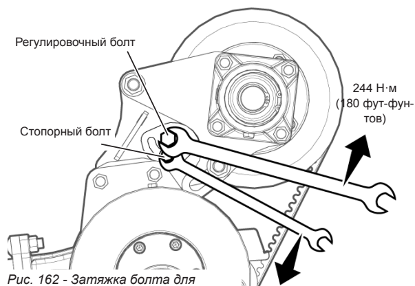
Рис. 162 - Затяжка болта для натяжения ремня.
