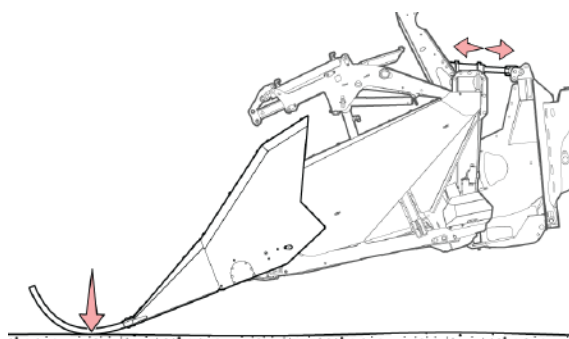
Рис. 65 - Жатка наклонена наружу, делители касаются земли
