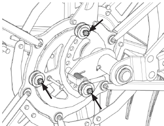
Рис. 212 - Уплотнительные кольца мотовила
