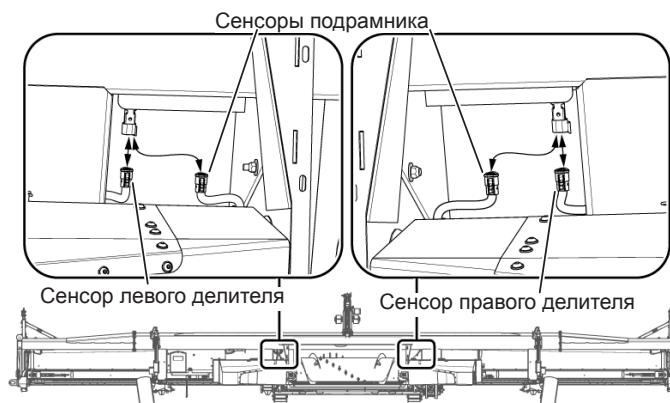
Рис. 126 - Выбор сенсоров при работе в режиме жесткой жатки
