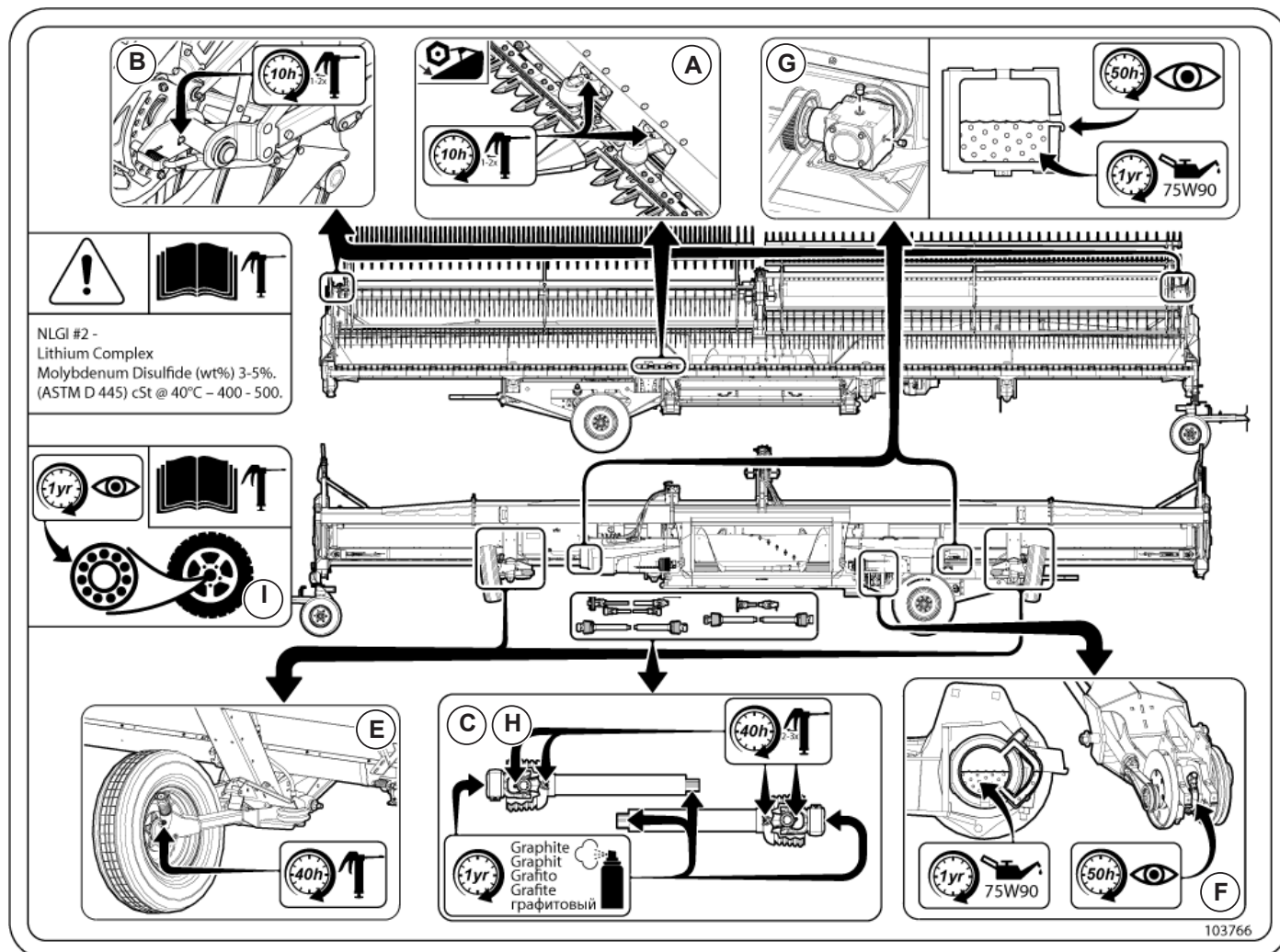
Рис. 278 - Места расположения точек нанесения смазки.
