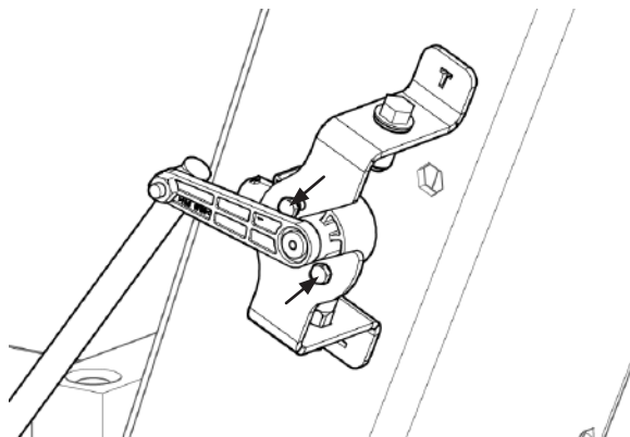
Рис. 267 - Регулировка сенсора контроля высоты жатки
