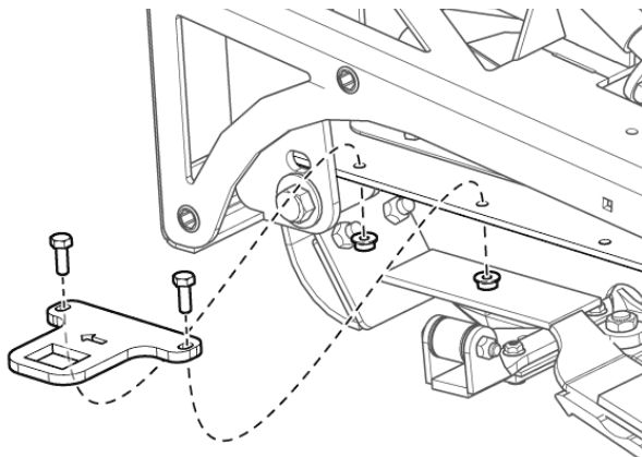
Рис. 98 - Установите стопорную пластину
