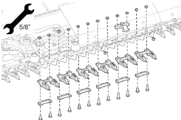
Рис. 229 - Снятие защитных устройств, которые окружают головку левого ножа
