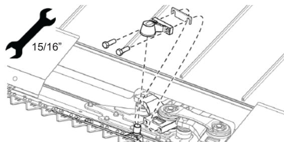
Рис. 227 - Снятие корпуса подшипников с головки правого ножа
