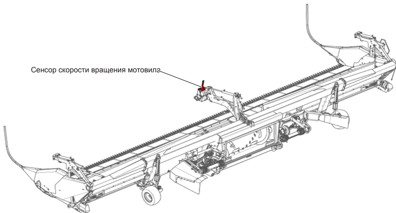
Рис. 308 - Расположение сенсора скорости.
