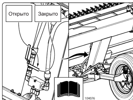
Рис. 68 - Запорный клапан копирующего колеса
