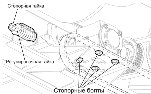
Рис. 156 - Регулировка натяжения второго приводного ремня левого полотенного транспортера.
