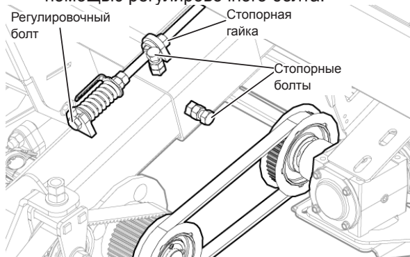
Рис. 176 - Снятие первого ремня правого полотенного транспортера для получения доступа к приводному ремню
