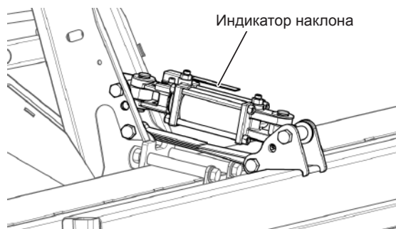
Рис. 110 - Гидравлический цилиндр и индикатор наклона
