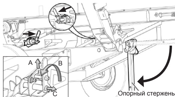
Рис. 49 - Разблокировка транспортного комплекта и опускание опорного стержня.
