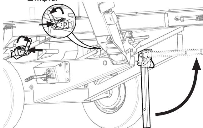
Рис. 285 - Прикрепление транспортной тележки к жатке.
