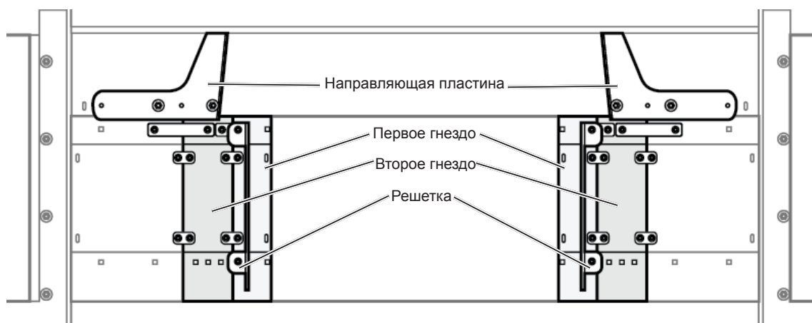
Рис. 295 - Гнезда AGCO.
