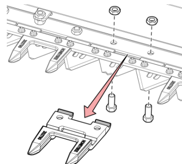
Рис. 234 - Снятие сдвоенный палец
