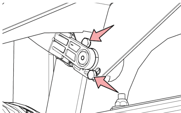
Рис. 271 - Регулировка сенсора подрамника
