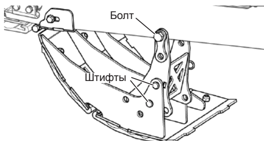
Рис. 85 - Положение 4: большая высота среза, ~8 дюймов (20 см)
