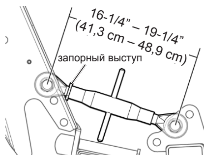
Рис. 258 - Сведения о верхнем звене
