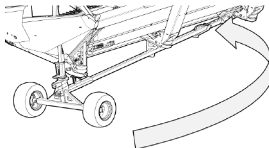
Рис. 289 - Поворот сцепного стержня в положение для хранения.
