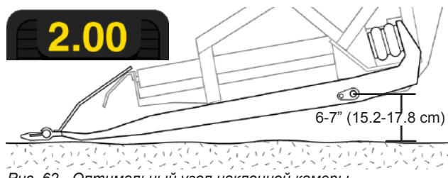
Рис. 62 - Оптимальный угол наклонной камеры.
