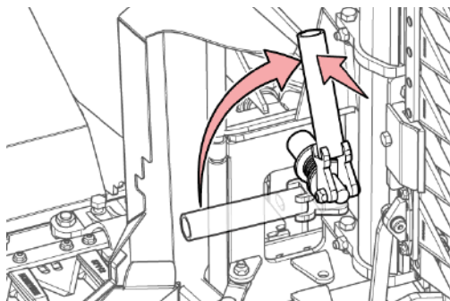
Рис. 105 - Зафиксируйте узел вертикальных ножниц с помощью стопорного рычага
