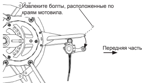
Рис. 283 - Опускание пальцев мотовила для транспортировки
