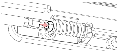
Рис. 187 - Затяните гайку
