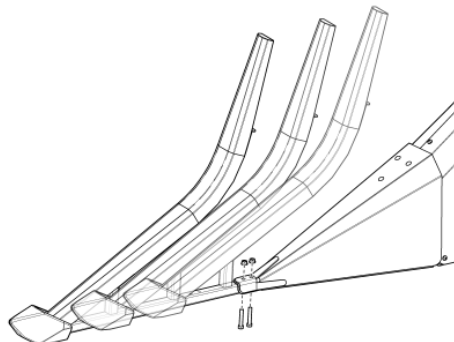
Рис. 119 - Насадки для боковых делителей
