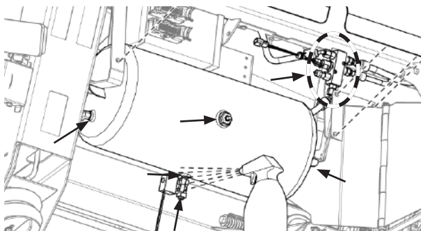
Рис. 272 - Проверка ресивера на предмет утечек.
