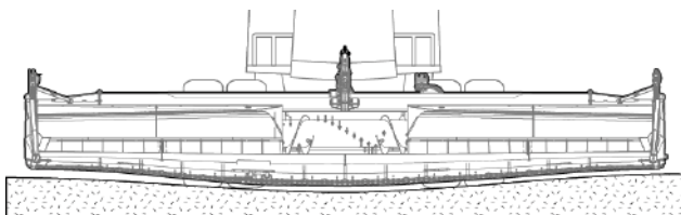
Рис. 120 - Режим гибкой жатки.
