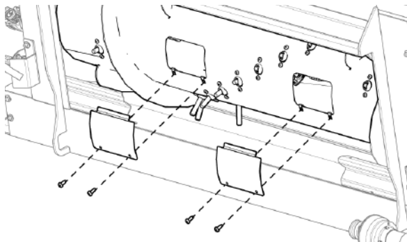
Рис. 255 - Доступ к внутренней части барабана подающего шнека
