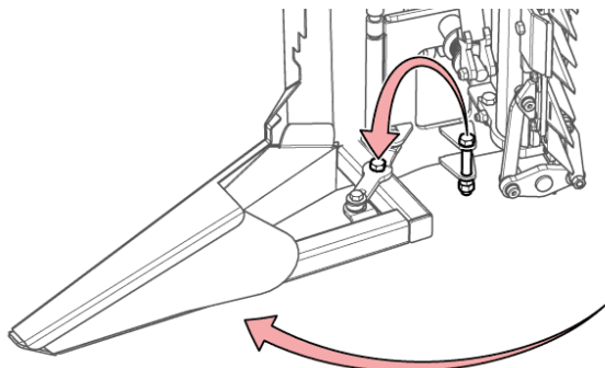
Рис. 102 - Зафиксируйте вертикальные ножницы в открытом положении
