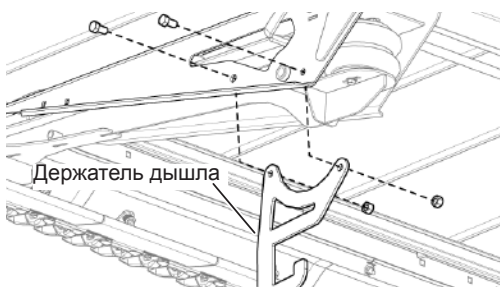
Рис. 47 - Снятие держателя дышла передней тележки
