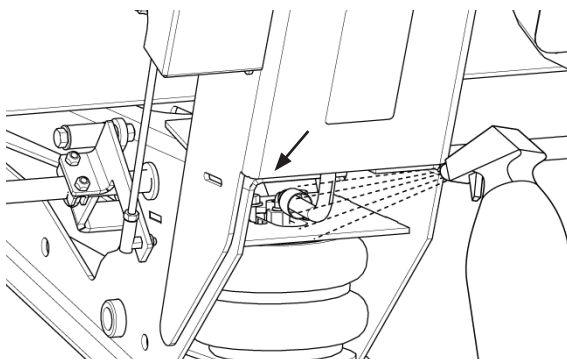
Рис. 274 - Проверка фитингов пневматических подушек на предмет утечек.
