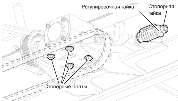
Рис. 160 - Регулировка натяжения второго ремня правого полотенного транспортера
