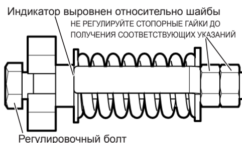
Рис. 151 - Положение индикатора натяжения.
