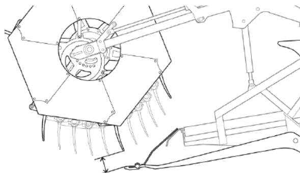
Рис. 72 - Расстояние между пальцами мотовила и режущим аппаратом.
