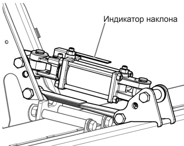
Рис. 259 - Гидравлический цилиндр наклона
