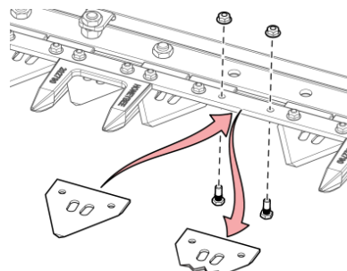
Рис. 235 - Замена режущего сегмента
