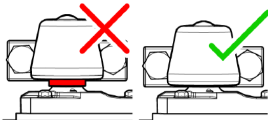
Рис. 232 - Проверка правильности установки корпуса подшипников
