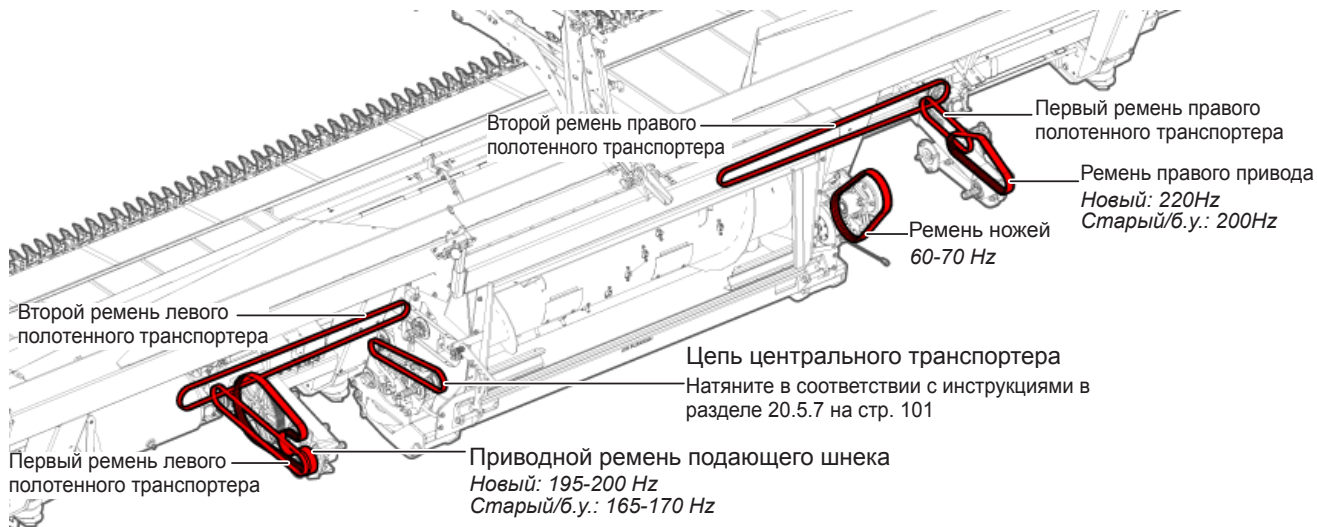
Рис. 150 - Места расположения приводных ремней
