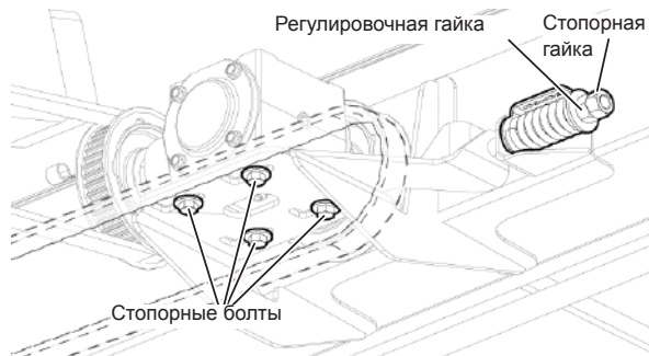
Рис. 177 - Регулировка натяжения второго ремня правого полотенного транспортера.
