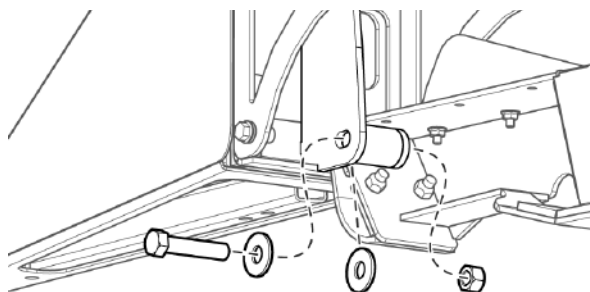
Рис. 116 - Положения блокировки делителей
