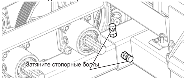
Рис. 170 - Стопорные болты первого приводного ремня левого полотенного транспортера.
