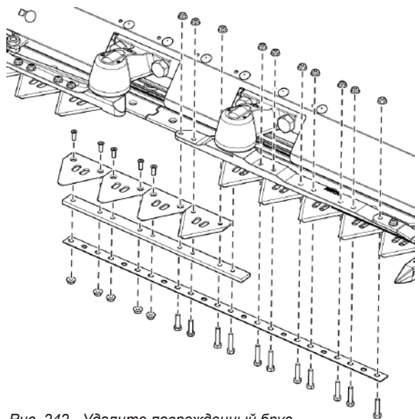
Рис. 242 - Удалите поврежденный брус перекрытия
