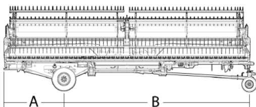
Рис. 279 - Размеры прицепа
