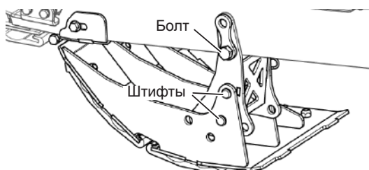
Рис. 84 - Положение 3: умеренно высокая высота среза
